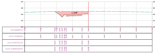
SECCION TRANSVERSAL PROG.: 9+066.50
