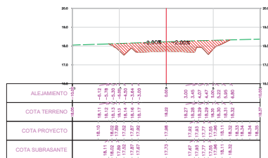
SECCION TRANSVERSAL PROG.: 0+350.00
