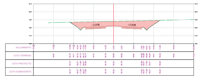
SECCION TRANSVERSAL PROG.: 94575.00
