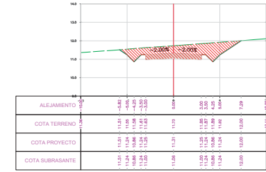
SECCION TRANSVERSAL PROG.: 0+975.00
