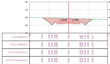
SECCION TRANSVERSAL PROG.: 9+175.00
