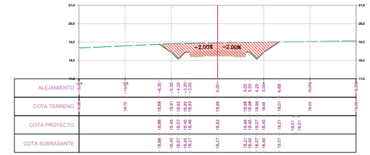
SECCION TRANSVERSAL PROG: 6+043.33
