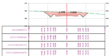
SECCION TRANSVERSAL PROG.: 0+335.00
