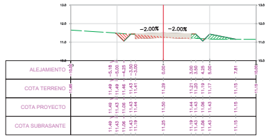
SECCION TRANSVERSAL PROG.: 9+295.00
