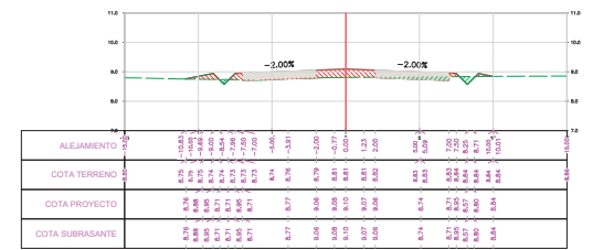
SECCION TRANSVERSAL PROG.: 9-495.80
