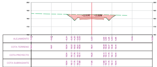
SECCION TRANSVERSAL PROG.: 9+238.00
