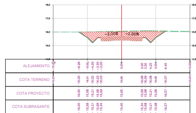
SECCION TRANSVERSAL PROG.: 0+200.00
