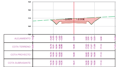
SECCION TRANSVERSAL PROG.: 9+125.00
