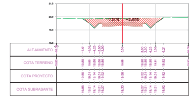
SECCION TRANSVERSAL PROG.: 0+175.00
