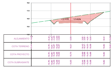
SECCION TRANSVERSAL PROG.: 9+925.00
