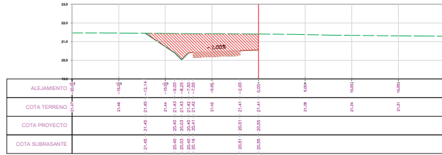
SECCION TRANSVERSAL PROG.: 9+059.50
