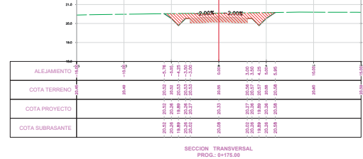
SECCION TRANSVERSAL PROG: 6+175.00
