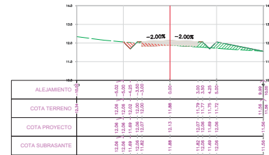
SECCION TRANSVERSAL PROG.: 9+182.05
