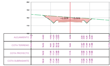
SECCION TRANSVERSAL PROG.: 0+1025.00
