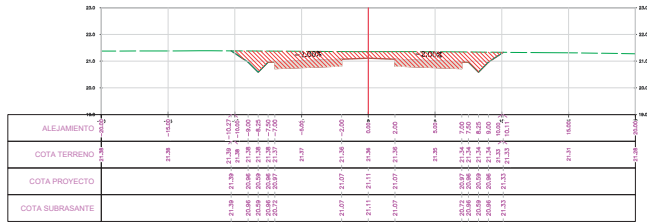
SECCION TRANSVERSAL PROG: 0+030.00
