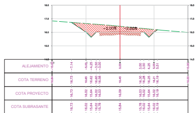
SECCION TRANSVERSAL PROG.: 0+1075.00
