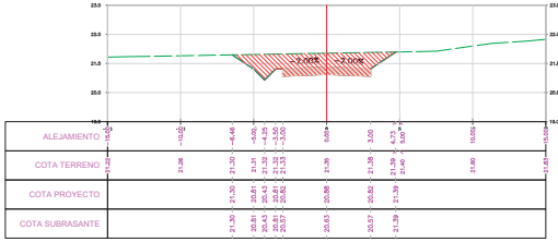
SECCION TRANSVERSAL PROG.: 9+156.00
