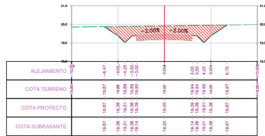
SECCION TRANSVERSAL PROG.: 0+190.00
