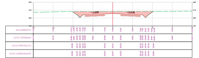
SECCION TRANSVERSAL PROG: 0+051.30
