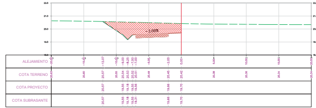
SECCION TRANSVERSAL PROG.: 9+075.50
