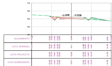
SECCION TRANSVERSAL PROG.: 0+1100.00
