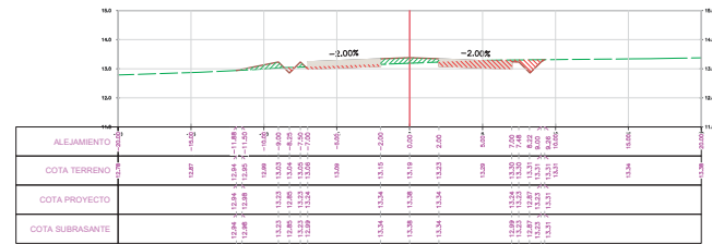
SECCION TRANSVERSAL PRG.: 9-275.00
