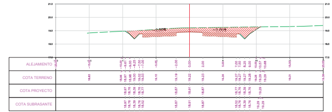
SECCION TRANSVERSAL PROG.: 94475.00
