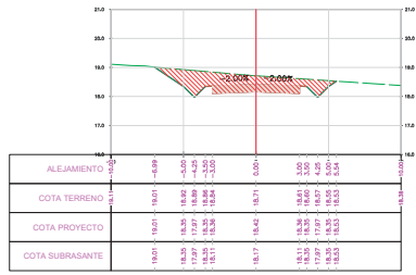
SECCION TRANSVERSAL PROG.: 0+1005.00
