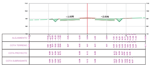
SECCION TRANSVERSAL PROG.: 9-448.73
