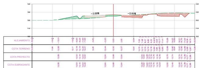
SECCION TRANSVERSAL PRG.: 9-350.00
