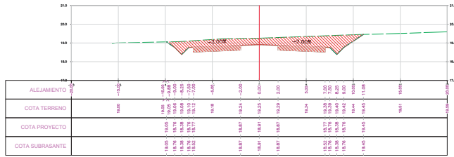
SECCION TRANSVERSAL PROG.: 94505.00
