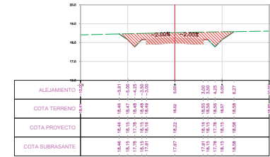
SECCION TRANSVERSAL PROG.: 0+325.00
