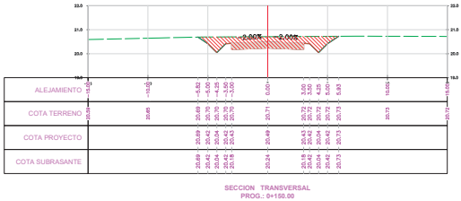
SECCION TRANSVERSAL PROG: 6+150.00
