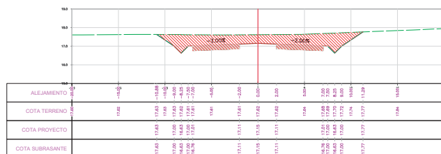
SECCION TRANSVERSAL PROG.: 9+159.50
