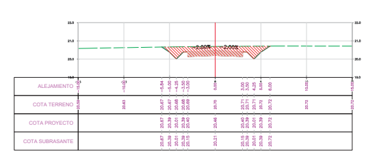
SECCION TRANSVERSAL PROG: 6+125.00
