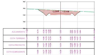
SECCION TRANSVERSAL PROG.: 9+200.00
