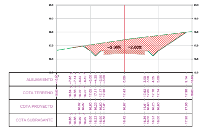
SECCION TRANSVERSAL PROG.: 9+947.98
