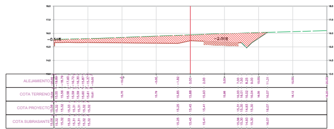
SECCION TRANSVERSAL PRG.: 9-200.00
