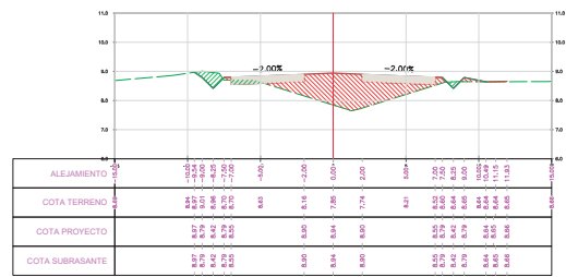
SECCION TRANSVERSAL PROG.: 9-473.81
