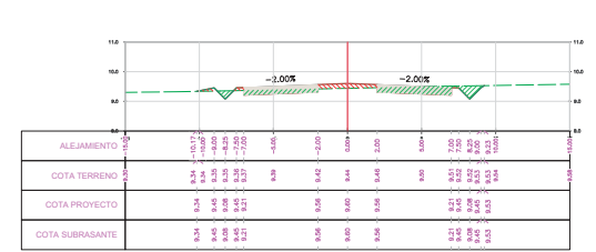
SECCION TRANSVERSAL PROG.: 9-429.60
