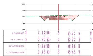
SECCION TRANSVERSAL PROG.: 9+422.50
