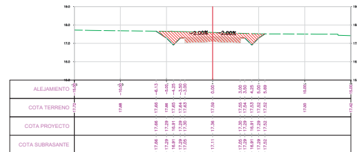
SECCION TRANSVERSAL PROG.: 9+314.17
