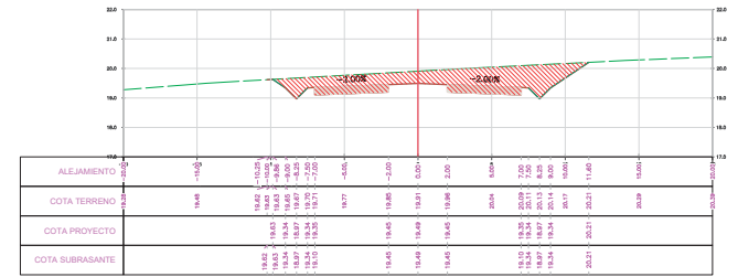
SECCION TRANSVERSAL PROG: 0+116.55
