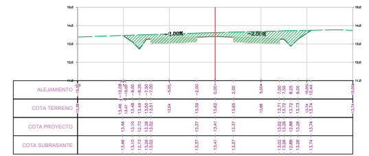
SECCION TRANSVERSAL PROG.: 9-331.14
