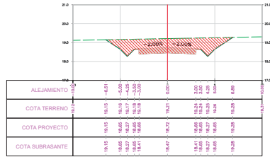
SECCION TRANSVERSAL PROG.: 0+280.00
