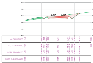
SECCION TRANSVERSAL PROG.: 9+900.00
