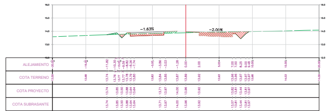
SECCION TRANSVERSAL PRG.: 9-200.00
