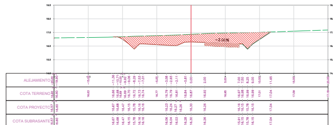
SECCION TRANSVERSAL PROG.: 9+175.50
