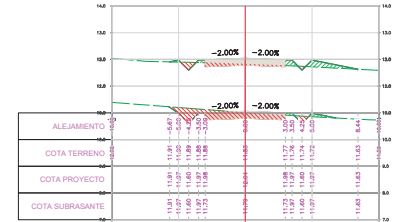
SECCION TRANSVERSAL PROG.: 9+118.15
