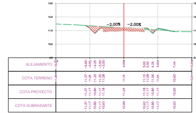
SECCION TRANSVERSAL PROG.: 9+100.00
