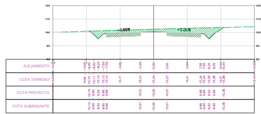
SECCION TRANSVERSAL PROG.: 9-433.10
