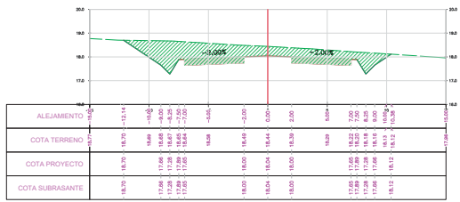
SECCION TRANSVERSAL PROG.: 9-267.45
