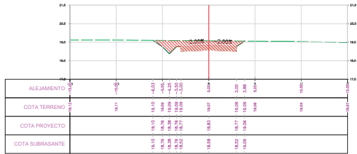
SECCION TRANSVERSAL PROG.: 9+250.00
