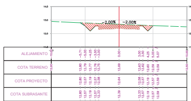
SECCION TRANSVERSAL PROG.: 9+250.00
