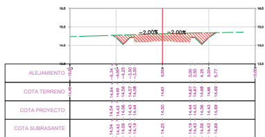
SECCION TRANSVERSAL PROG.: 0+395.67
