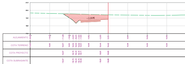
SECCION TRANSVERSAL PROG.: 9+109.50
