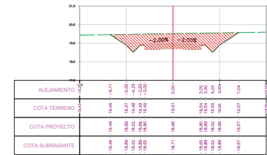
SECCION TRANSVERSAL PROG.: 0+250.00
