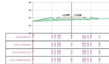
SECCION TRANSVERSAL PROG.: 0+1200.00
