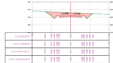
SECCION TRANSVERSAL PROG.: 9+225.00
