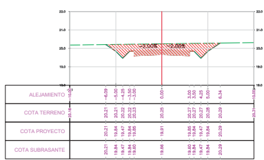
SECCION TRANSVERSAL PROG.: 9+400.00
