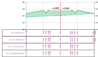
SECCION TRANSVERSAL PROG.: 0+1225.00
