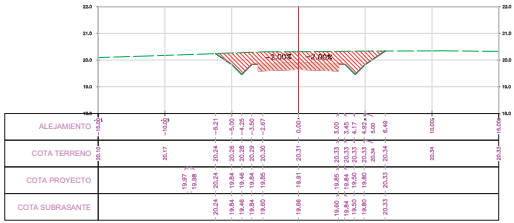
SECCION TRANSVERSAL PROG: 6+585.65
