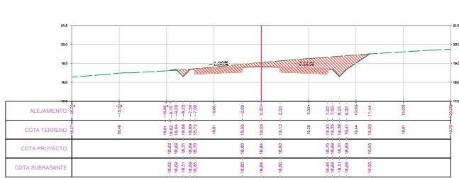
SECCION TRANSVERSAL PROG: 0+165.00
