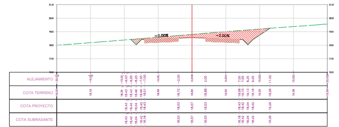
SECCION TRANSVERSAL PROG: 0+185.90
