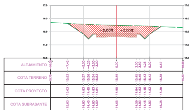
SECCION TRANSVERSAL PROG.: 0+305.00
