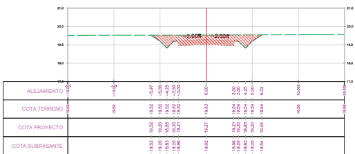
SECCION TRANSVERSAL PROG: 6+250.00
