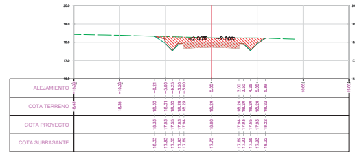
SECCION TRANSVERSAL PROG.: 9+255.99
