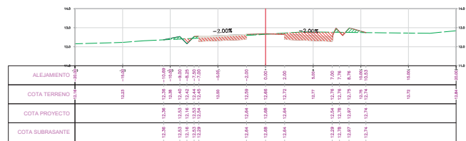
SECCION TRANSVERSAL PRG.: 9-300.00
