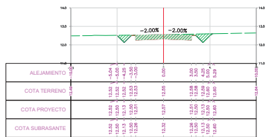
SECCION TRANSVERSAL PROG.: 0+250.00
