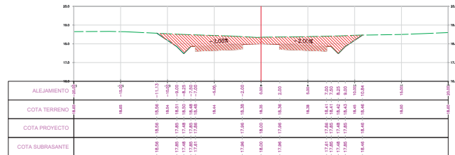
SECCION TRANSVERSAL PROG.: 9+125.50
