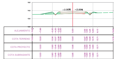
SECCION TRANSVERSAL PROG.: 0+1185.00
