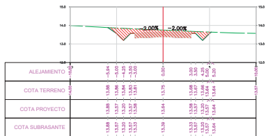
SECCION TRANSVERSAL PROG.: 0+245.45
