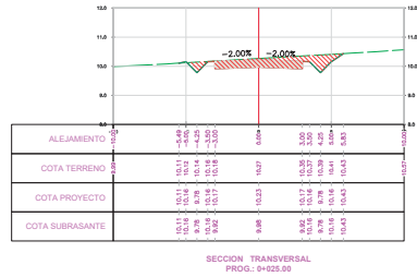
SECCION TRANSVERSAL PROG.: 0+925.00
