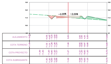
SECCION TRANSVERSAL PROG.: 9+145.00
