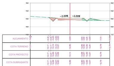
SECCION TRANSVERSAL PROG.: 0+223.00
