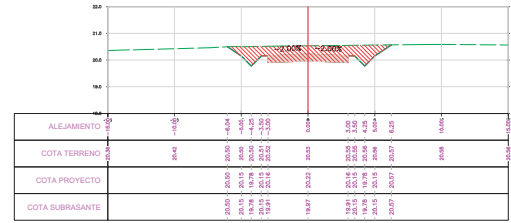
SECCION TRANSVERSAL PROG: 6+100.00
