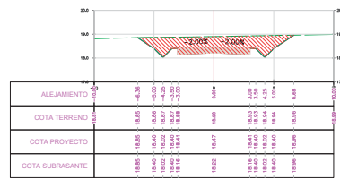
SECCION TRANSVERSAL PROG.: 0+300.00
