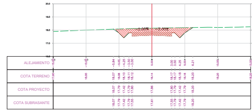
SECCION TRANSVERSAL PROG: 6+025.00
