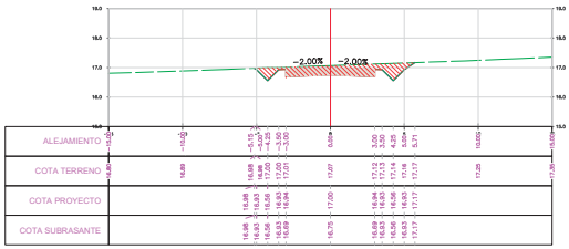
SECCION TRANSVERSAL PROG: 6+000.00
