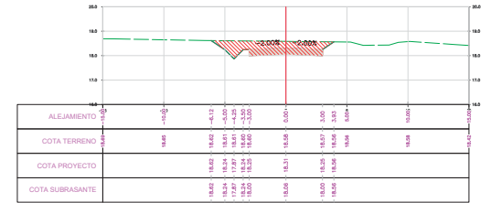
SECCION TRANSVERSAL PROG.: 9+275.00
