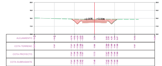
SECCION TRANSVERSAL PROG.: 9+277.52
