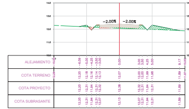
SECCION TRANSVERSAL PROG.: 9+105.00
