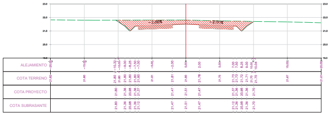
SECCION TRANSVERSAL PROG: 0+015.00
