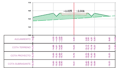
SECCION TRANSVERSAL PROG.: 0+1250.00
