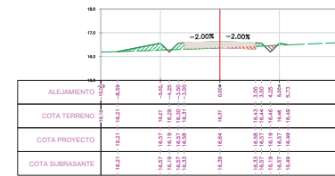
SECCION TRANSVERSAL PROG.: 0+1275.00
