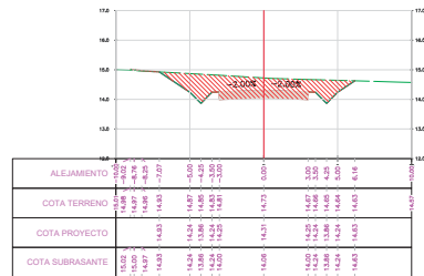
SECCION TRANSVERSAL PROG.: 0+275.00
