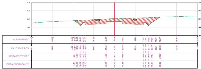
SECCION TRANSVERSAL PROG: 0+100.00
