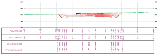
SECCION TRANSVERSAL PROG: 0+078.88
