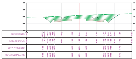
SECCION TRANSVERSAL PROG.: 9-275.68
