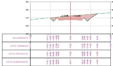
SECCION TRANSVERSAL PROG.: 9+100.00
