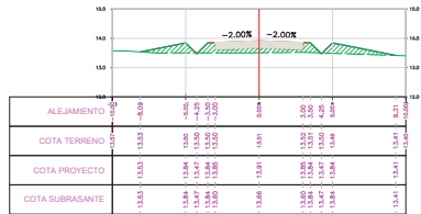
SECCION TRANSVERSAL PROG.: 0+1155.00
