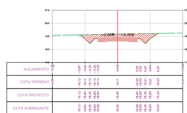
SECCION TRANSVERSAL PROG.: 9+522.00
