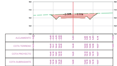
SECCION TRANSVERSAL PROG.: 9+150.00
