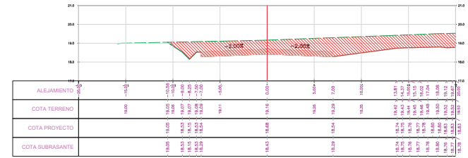
SECCION TRANSVERSAL PROG.: 94525.00
