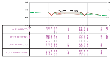
SECCION TRANSVERSAL PROG.: 9+015.51
