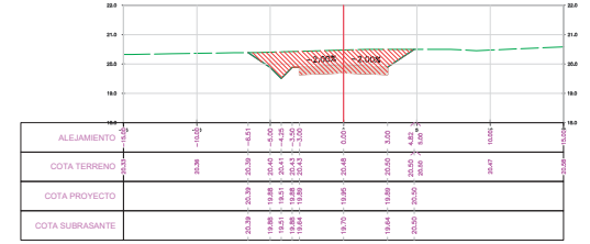
SECCION TRANSVERSAL PROG.: 9+195.00
