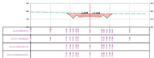
SECCION TRANSVERSAL PROG.: 9+295.00
