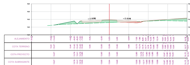
SECCION TRANSVERSAL PRG.: 9-375.00
