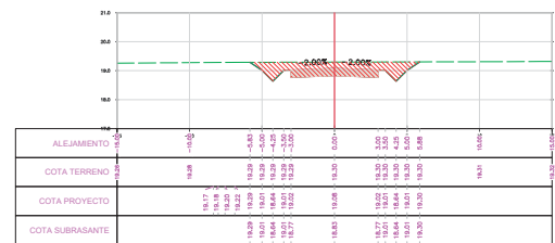
SECCION TRANSVERSAL PROG: 6+275.00
