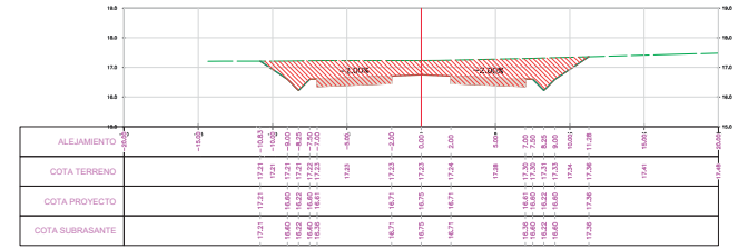
SECCION TRANSVERSAL PROG.: 94425.00
