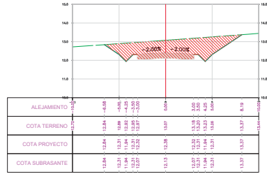
SECCION TRANSVERSAL PROG.: 0+980.00
