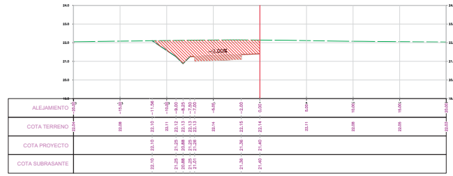
SECCION TRANSVERSAL PROG.: 9+025.50
