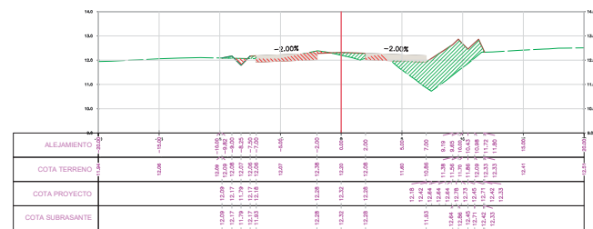
SECCION TRANSVERSAL PRG.: 9-325.00
