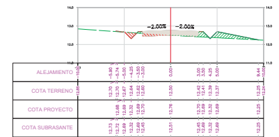
SECCION TRANSVERSAL PROG.: 9+299.05
