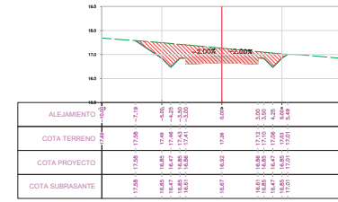
SECCION TRANSVERSAL PROG.: 0+1055.00
