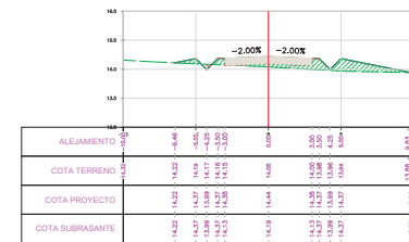
SECCION TRANSVERSAL PROG.: 0+1125.00
