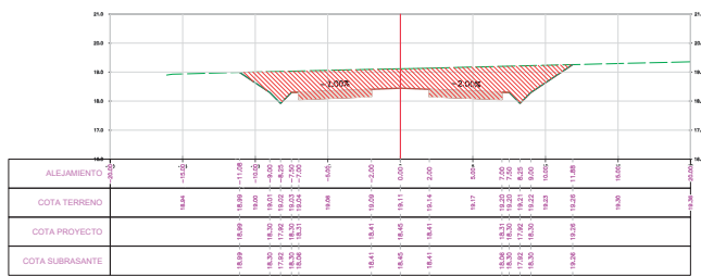
SECCION TRANSVERSAL PROG.: 94555.00
