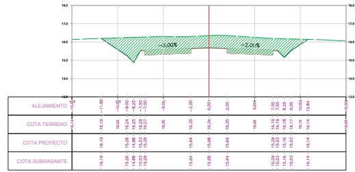
SECCION TRANSVERSAL PROG.: 9-304.20
